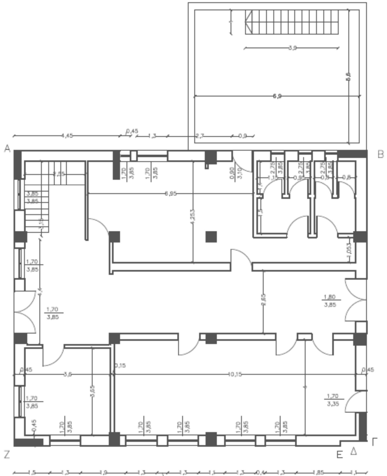
5.2. Κάτοψη Ισογείου κτιρίου Αναπτυξιακής Ροδότης Α.Ε. μετά την ανακαίνιση
